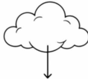
CUMULUS
